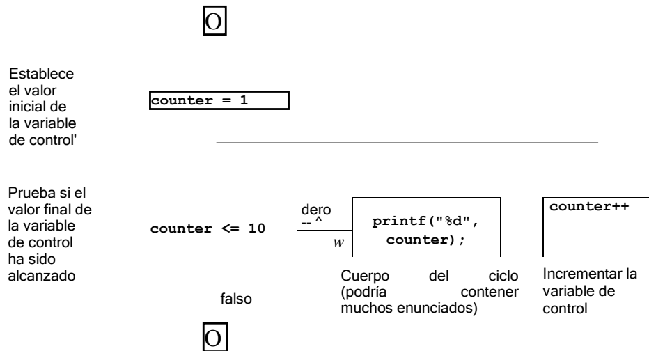
Fig. 4.4 Diagrama de flujo de una estructura for típica
