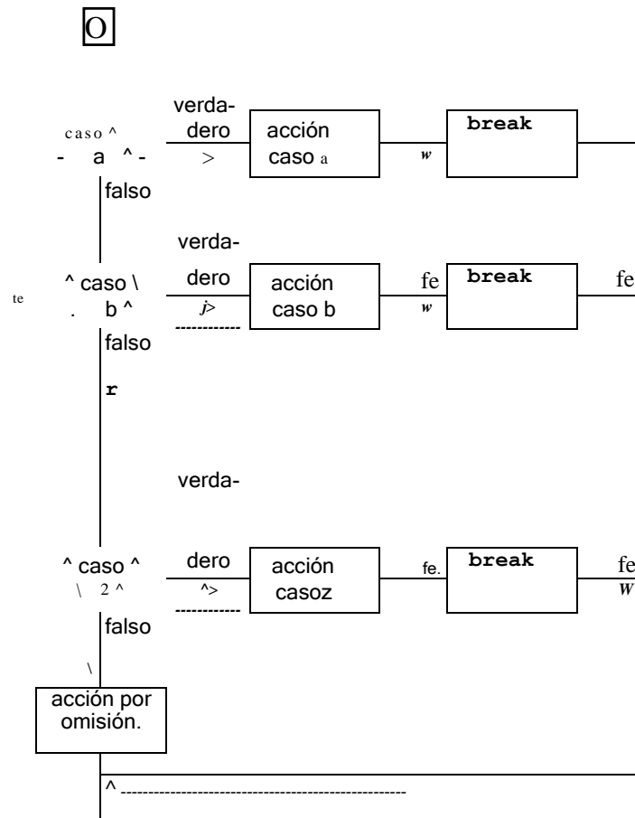
Fig. 4.8 La estructura de selección múltiple switch.
