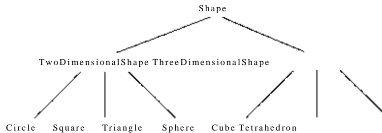
Fig. 19.3 Una porción de la jerarquía de clase Shape .
