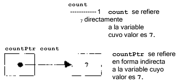
Fig. 7-1 Referenciación directa e Indirecta de una variable.
