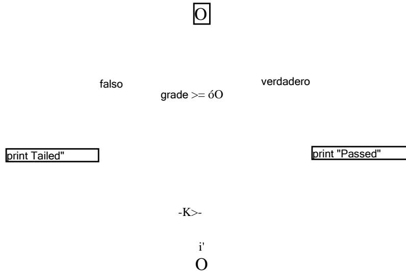
Fig. 3.3 Diagrama de flujo en C de la estructura de doble selección if/else .
