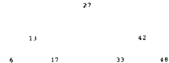
Fig. 12.21 Un árbol de búsqueda binario.
