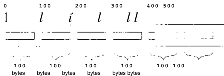
Fig. 11.10 Vista de un archivo de acceso directo con registros de longitud fija.
