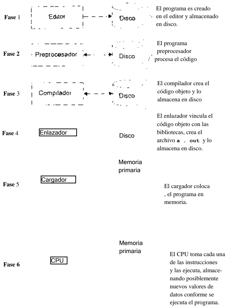
Fig. 1.1 Un entorno típico de C.
