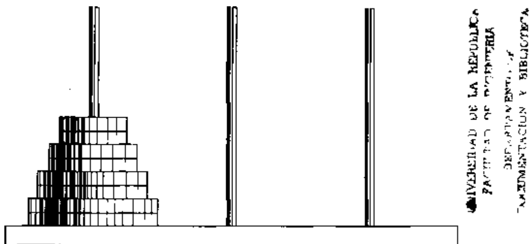
Fig. 5.18 Las Torres de Hanoi para el caso de cuatro discos.
