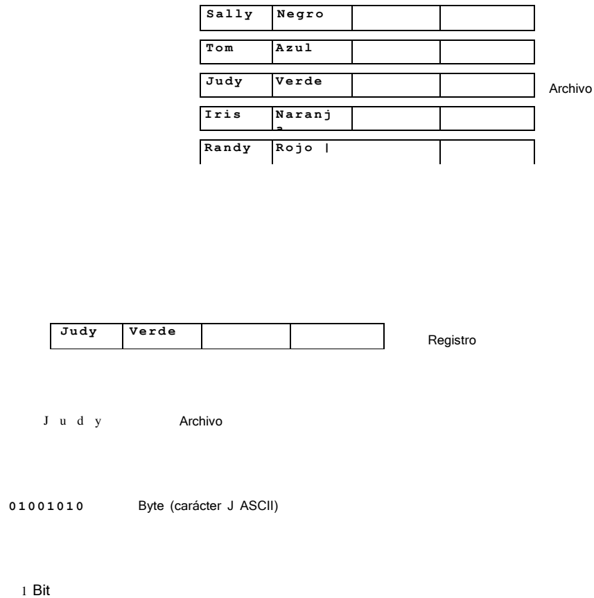
Fig. 11.1 La jerarquía de datos.
