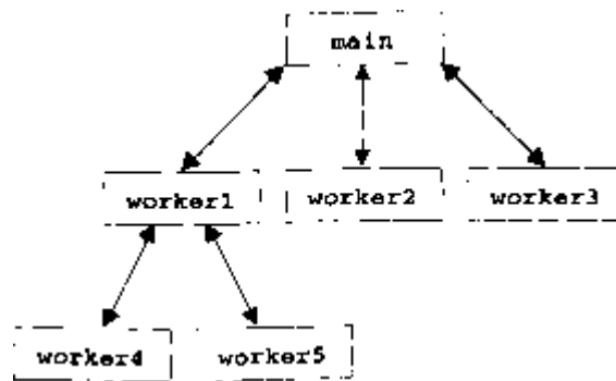
Fig. 5.1 Relación jerárquica función jefe/función trabajadora.
