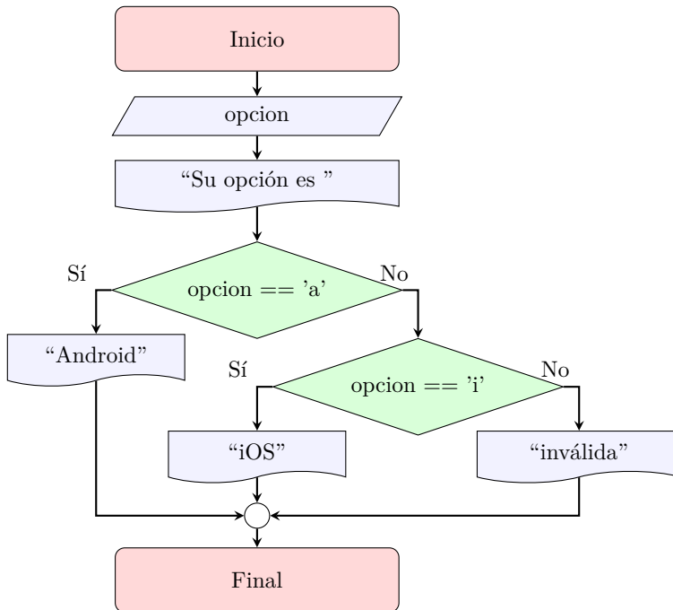
Figura 3.20: Diagrama de flujo del Algoritmo SistemaOperativo
