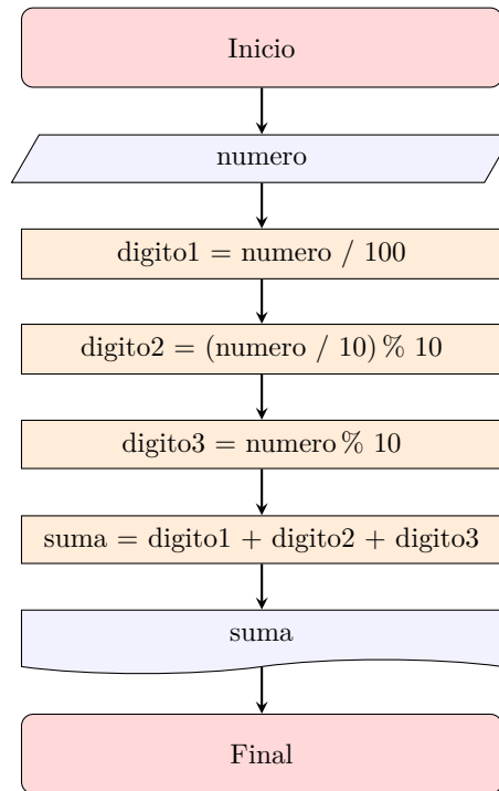
Figura 2.5: Diagrama de flujo del Algoritmo SumaDigitosNumero
