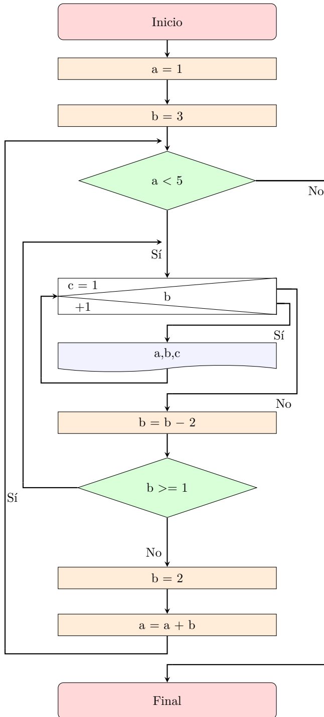
Figura 4.43: Diagrama de flujo del Algoritmo Tab1a2
